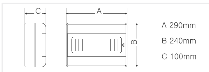
SCHEMA ESEMPIO – KOMBILUX 520, 1020 e 2040
