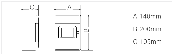
DIMENSIONI CENTRALINO SICURLUX 520, 1020 e 2040
