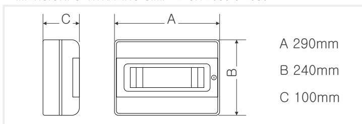
SCHEMA ESEMPIO – SIMPLELUX 520, 1020 e 2040
