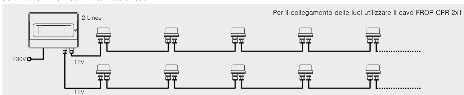
SCHEMA ESEMPIO – SIMPLELUX 2060 e 2080
