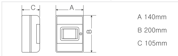
DIMENSIONI CENTRALINO SIMPLELUX 520, 1020 e 2040
